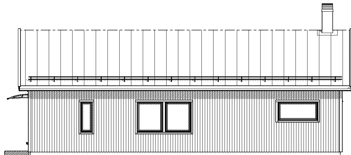
FASAD 1
