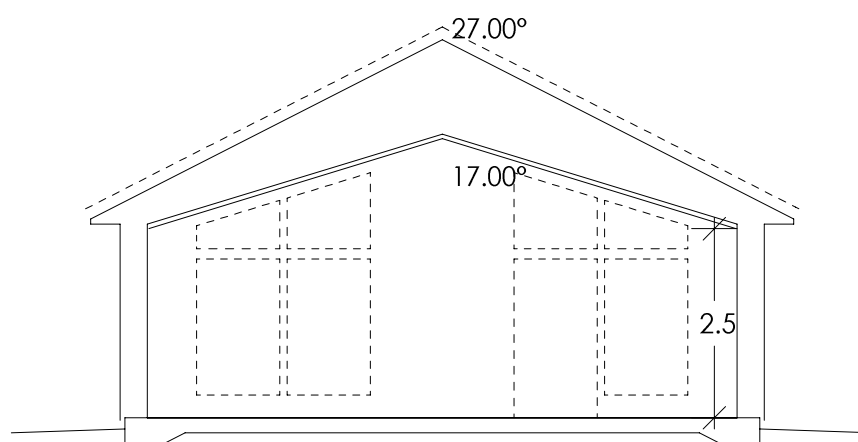
SEKTION B-B
