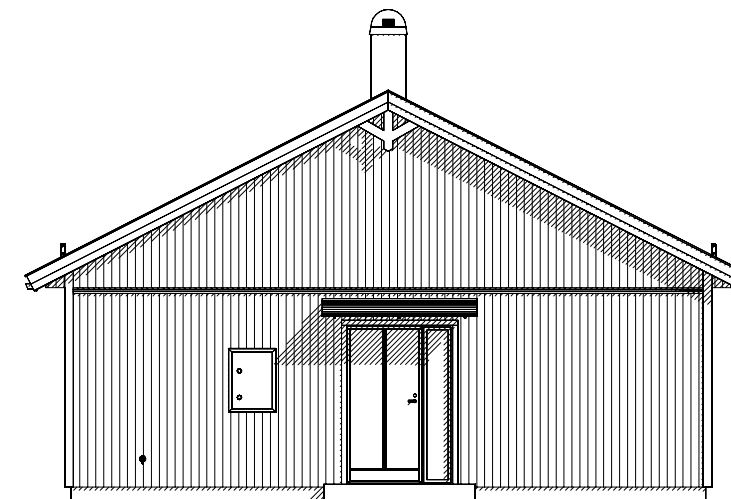
FASAD 4
