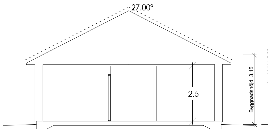
SEKTION A-A
