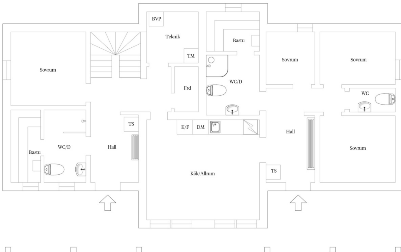
PLANSKISS ENTRÉPLAN
