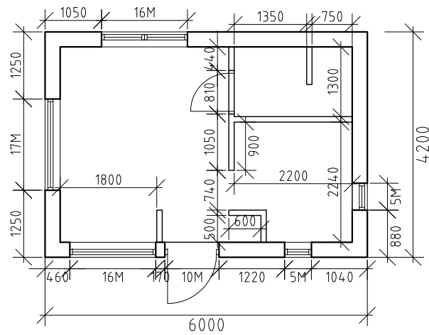
PLAN 1 MÅTTSÄTTNING
