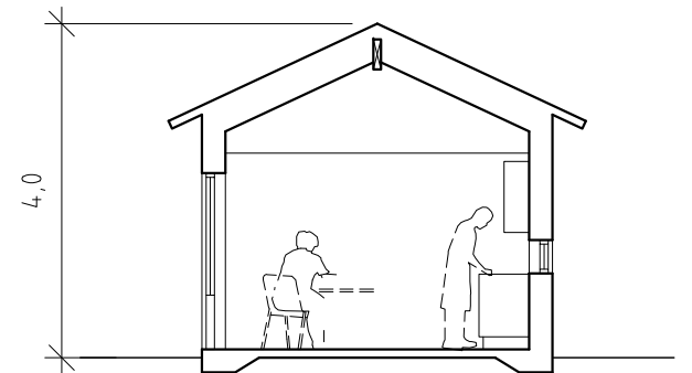
SEKTION B-B
